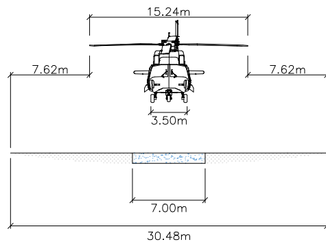
PISTA E ROTA DE TÁXI AÉREO – VISTA ESCALA 1:500
