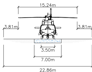
PISTA E ROTA DE TÁXI TERRESTRE – VISTA ESCALA 1:500
