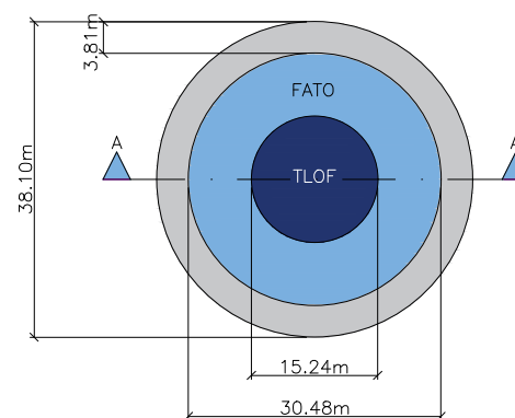
FATO E ÁREA DE SEGURANÇA ASSOCIADA – PLANTA ESCALA 1:1000
