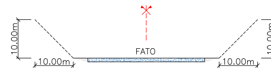
RAMPA LATERAL PROTEGIDA – CORTE AA ESCALA 1:1000
